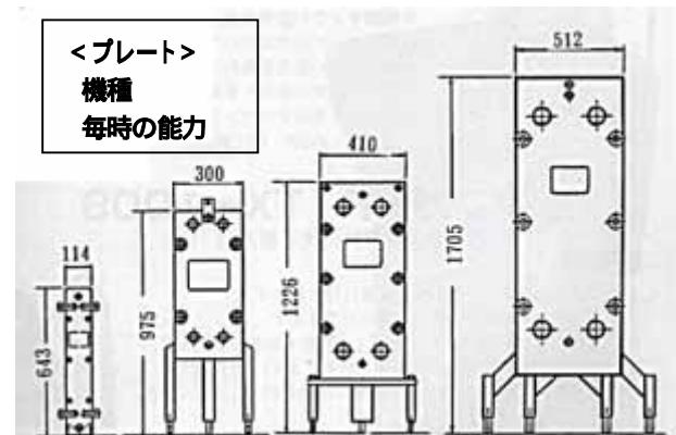
プレート機種: ジュニア型 SR-1 SR-2 SR-3 毎時の能力: 10~500L 500~5000L 5000~15000L 15000~30000L
